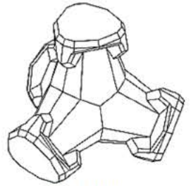
消波ブロック 意匠登録第1393309号
